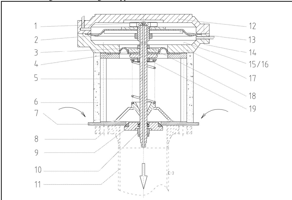
Ersatzteilzeichnung 1: Stellgerät Typ 86
