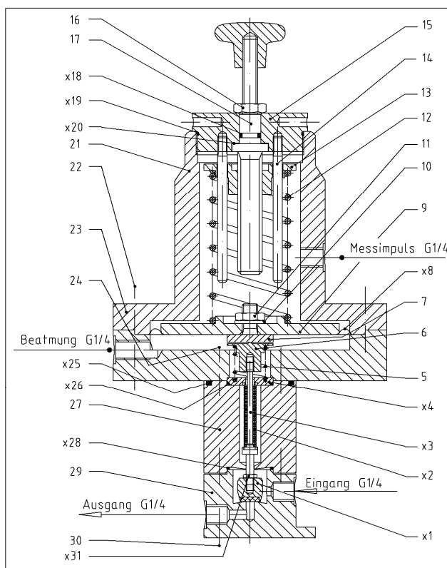
Ersatzteilzeichnung 2: Steuerregler Typ DUH
