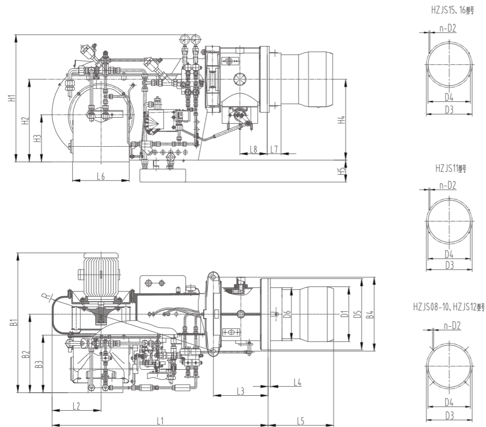
HZJS08-16 外形及开孔尺寸
